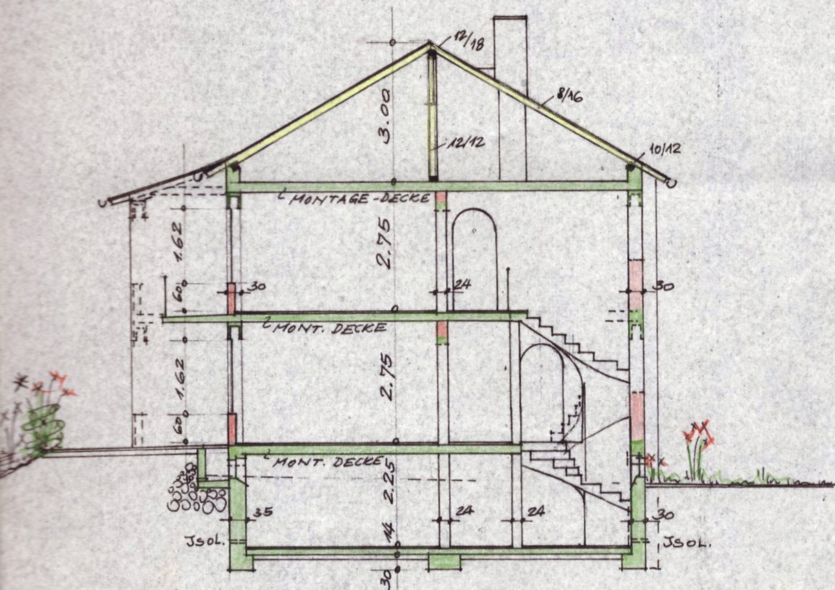
QUERSCHNITT M. 1 = 100
